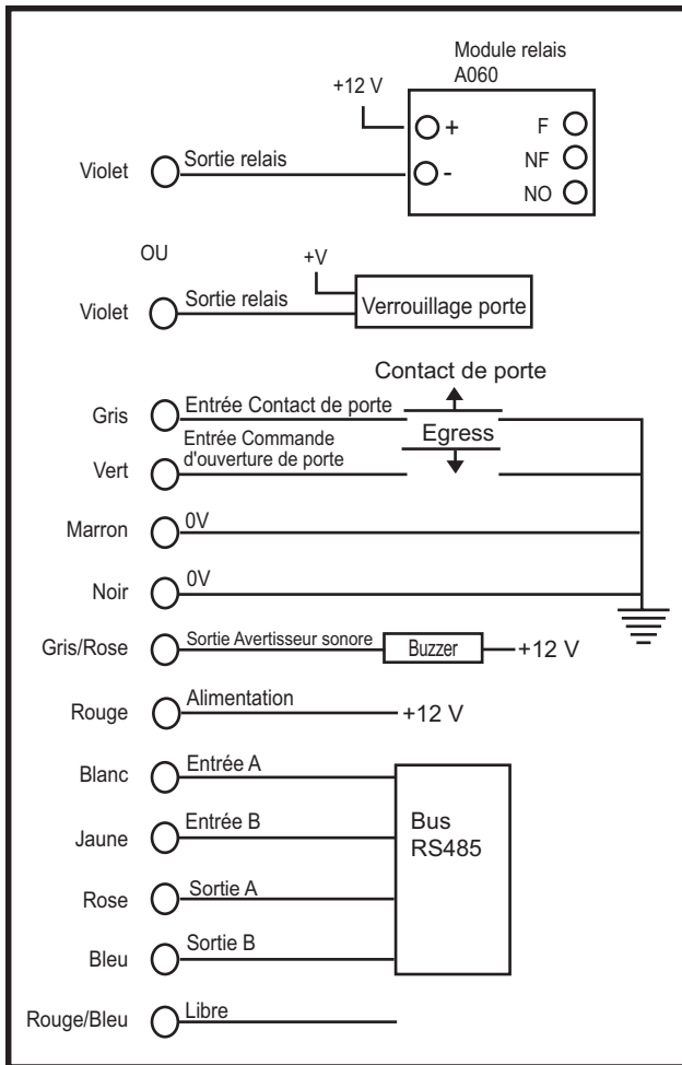
Raccordement en mode On-line
