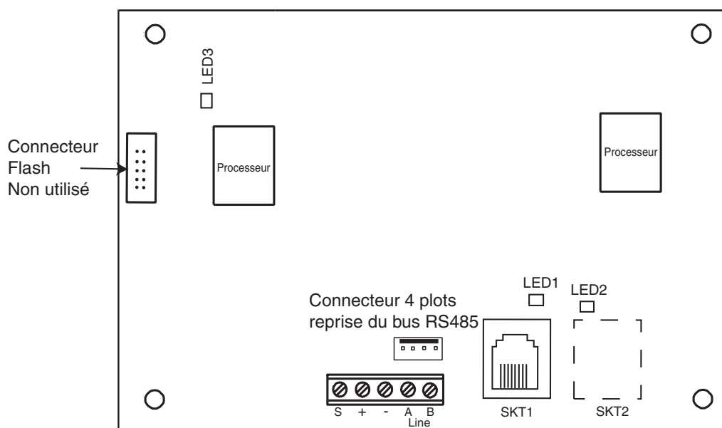
Carte électronique du module Ethernet
