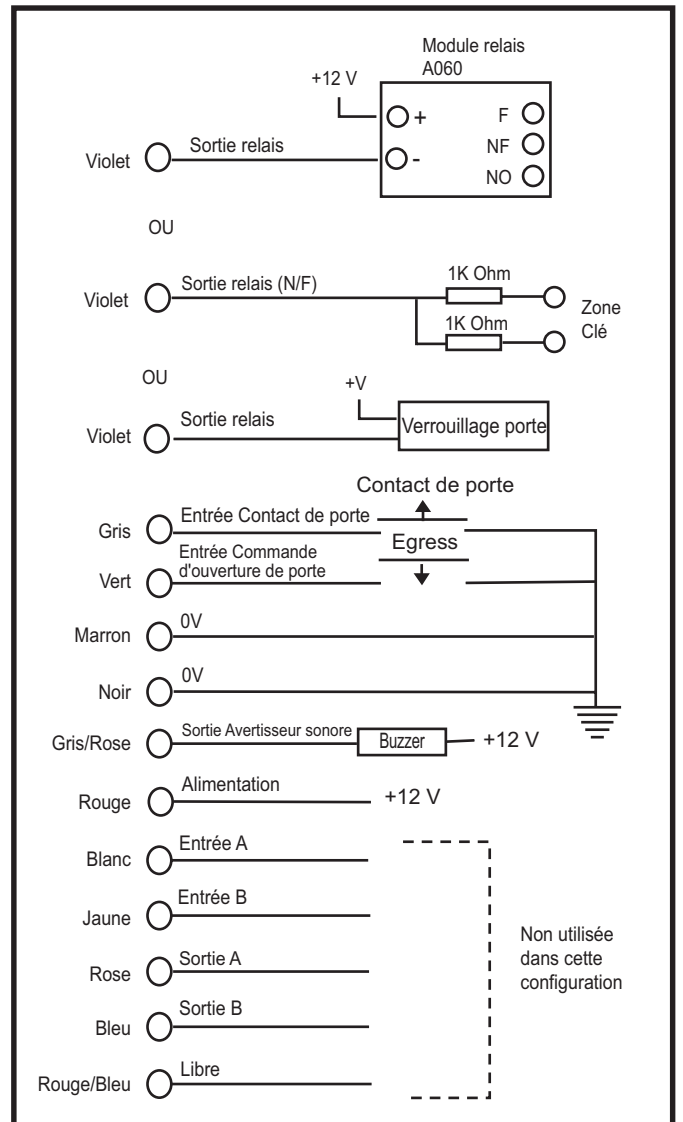
Raccordement en mode Autonome
