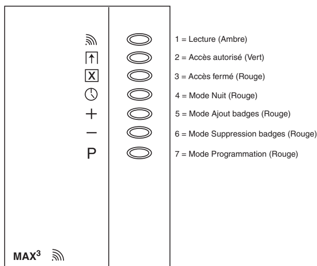
Voyants du MAX 3
