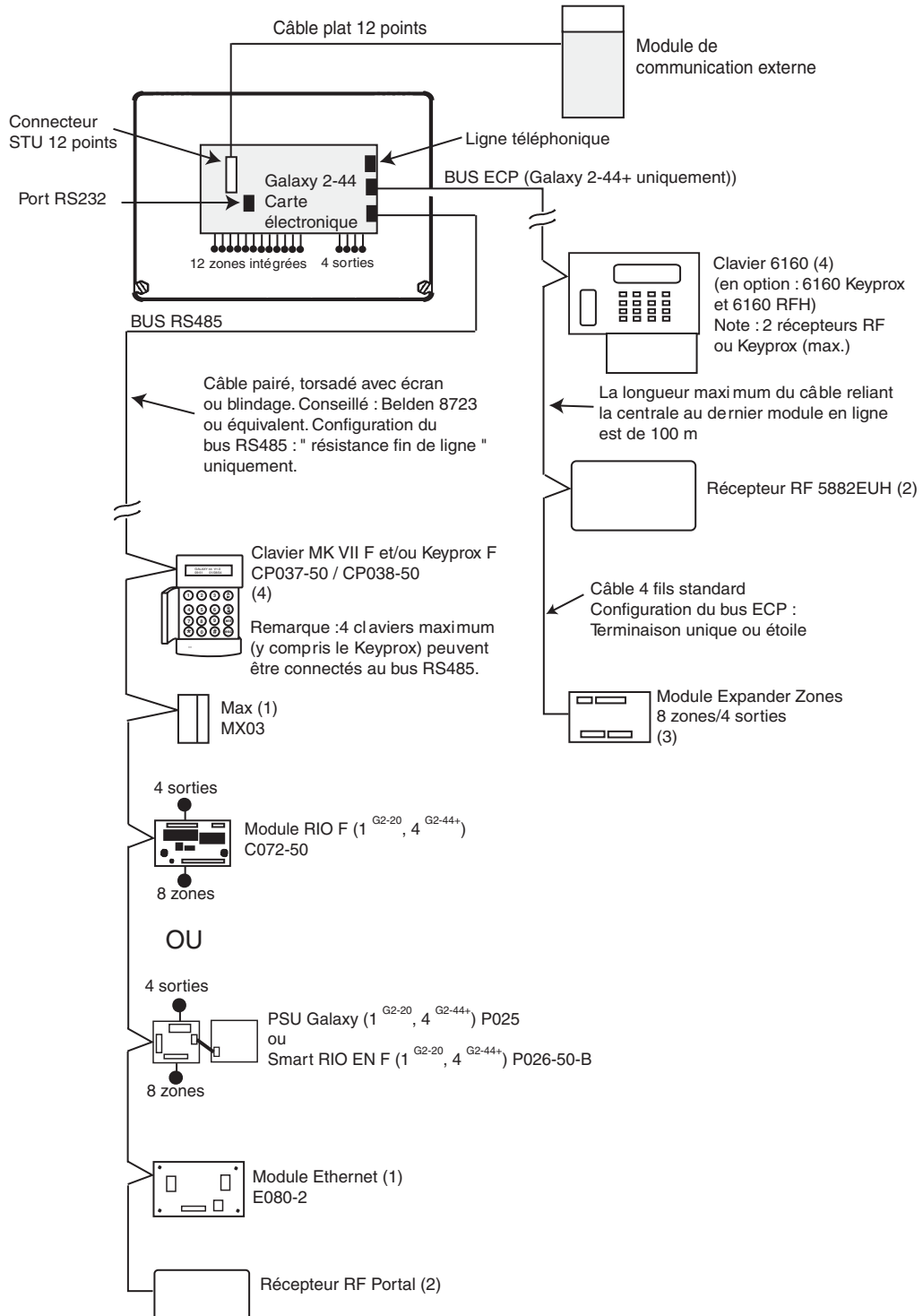
Architecture du système Galaxy 2
