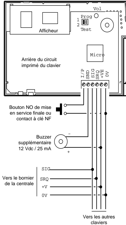
Figure 10. Raccordement d'un clavier 931
