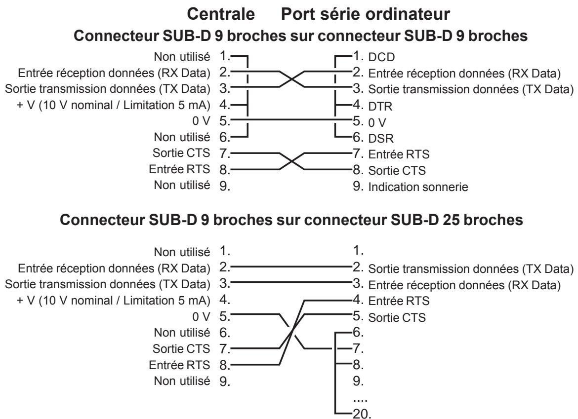
Figure 60. Signaux présents sur le connecteur série
