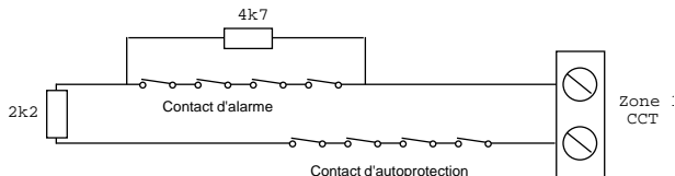
Figure 13. Raccordement de plusieurs contacts d'alarme avec autoprotection
