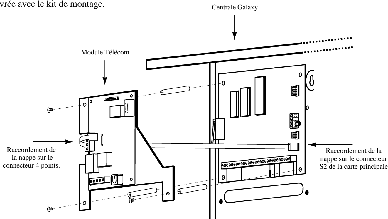
Figure 1-3. Raccordement du module Télécom F sur les centrales Galaxy 18/60 F.
